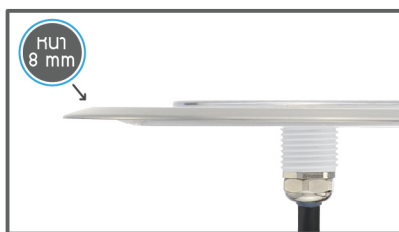
ตัวกรอบดวกรโคมใช้วัสดุ Stainless Steel 316 ความหนาเพียง 8 มิลลิเมตร
